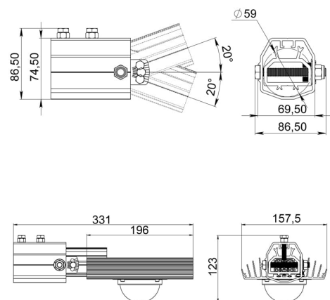
Габаритный чертеж
