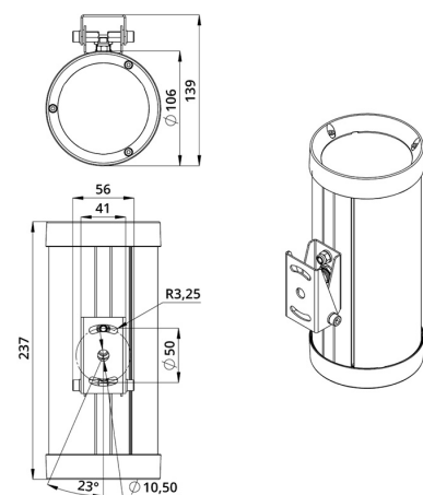
Габаритный чертеж
