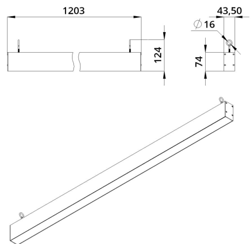
Габаритный чертеж
